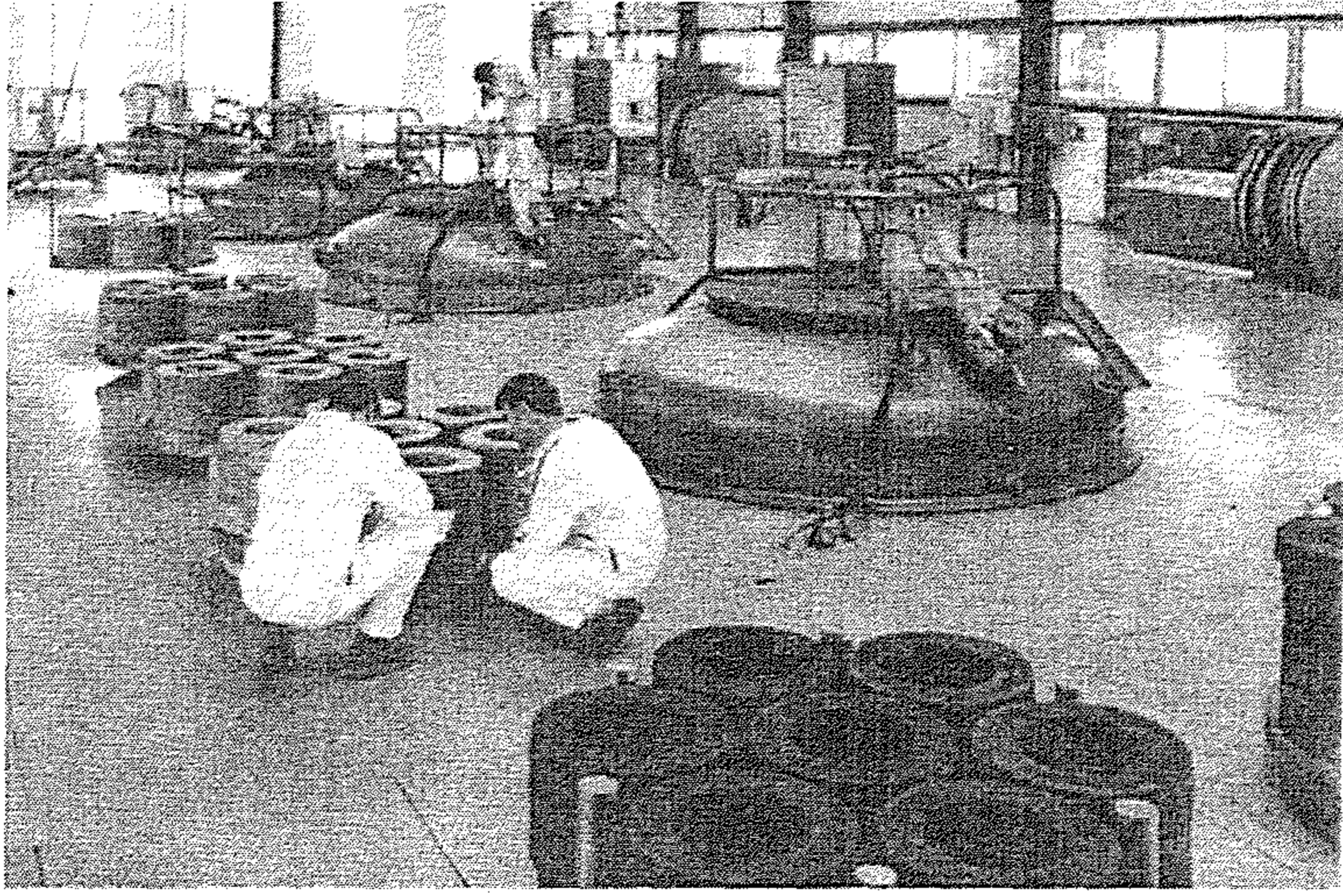
شكل ٣: معمل تكثيف
